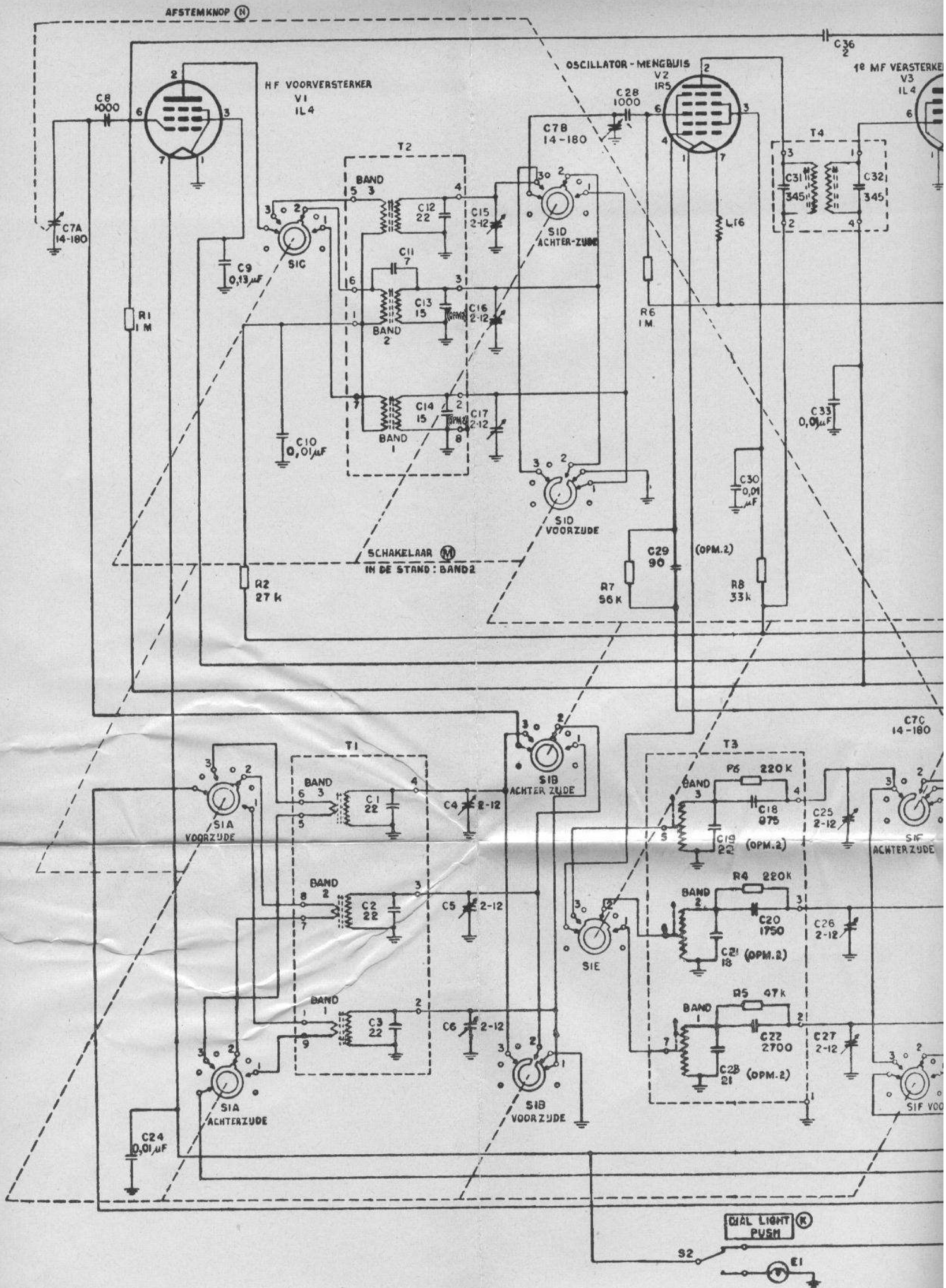
Fig. 74. Ontvangergedeelte van de Zend-ontvanger RT-77/G
