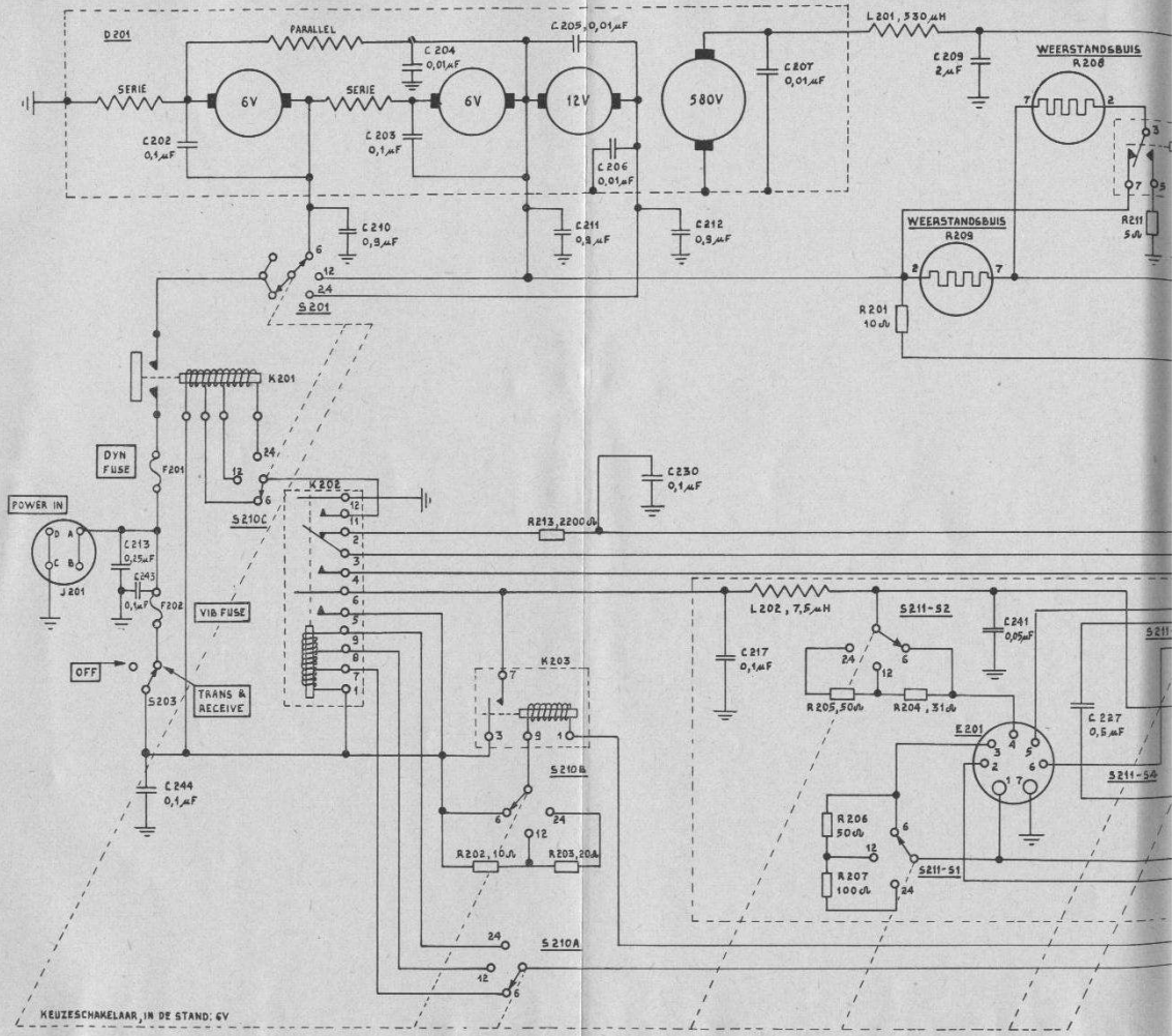
Fig. 77A. Voedingseenheid DY-88FR/GRC-9, prinseschema
