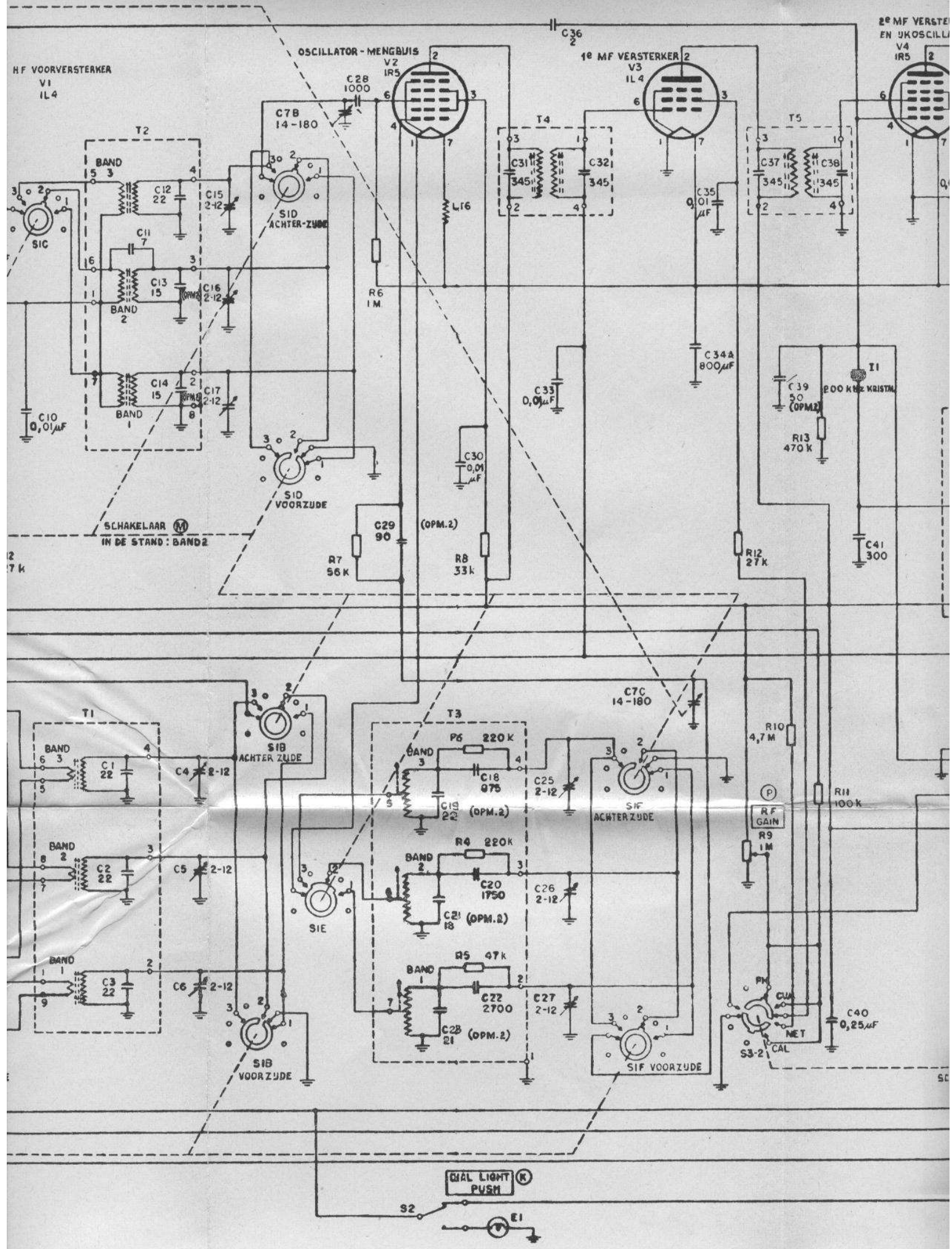
Fig. 74. Ontvangergedeelte van de Zend-ontvanger RT-77/GRC-9, prinsieschema
