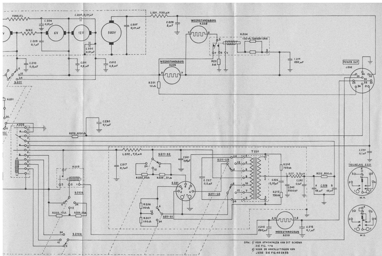
Fig. 77A. Voedingseenheid DY-88FR/GRC-9, prinsieschema
