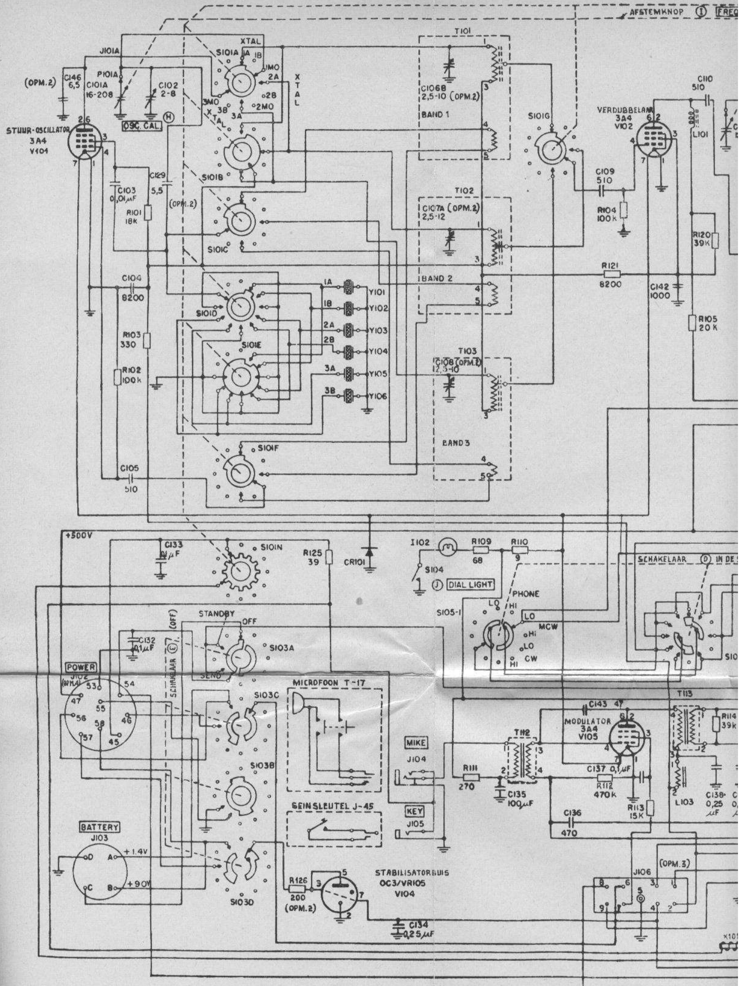
Fig. 75. Zendergedeelte van de Zend-ontvanger RT-77/GRC-9, pr
