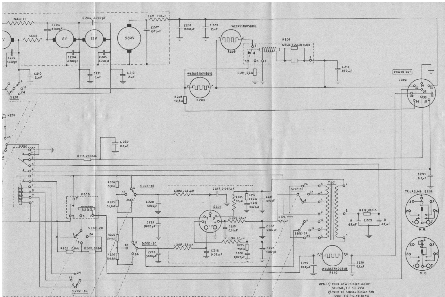
Fig. 77B. Voedingseenheid DY-88GY/GRC-9, prinseschema
