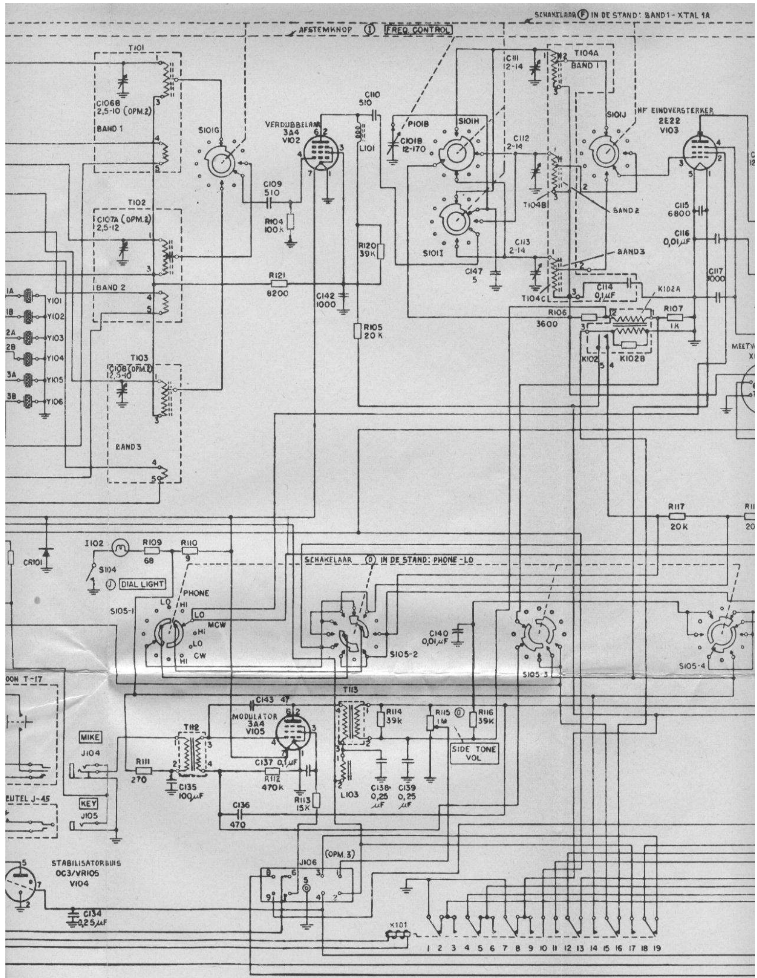
Fig. 75. Zendergedeelte van de Zend-ontvanger RT-77/GRC-9, prinseschema
